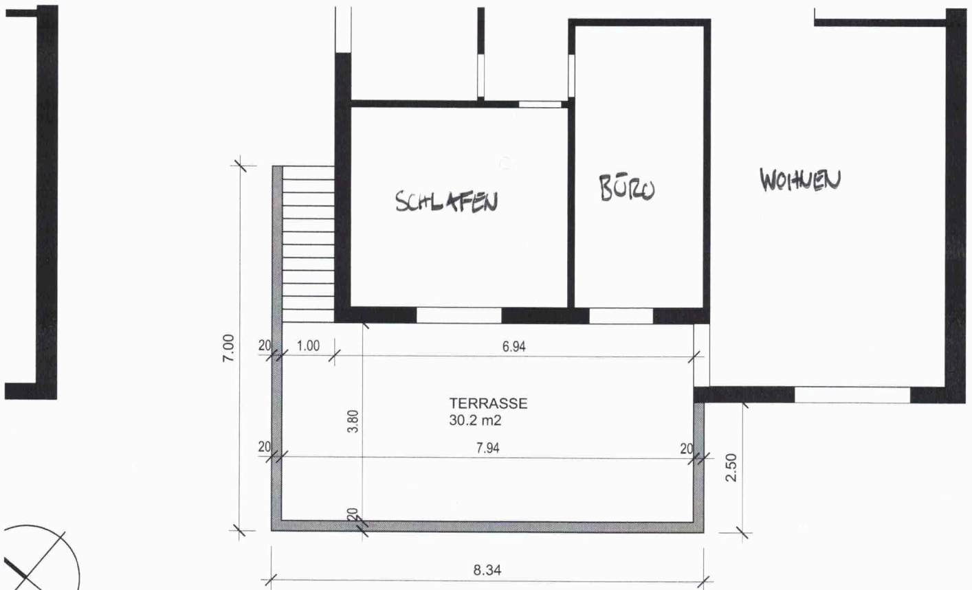
OBERGESCHOSS
