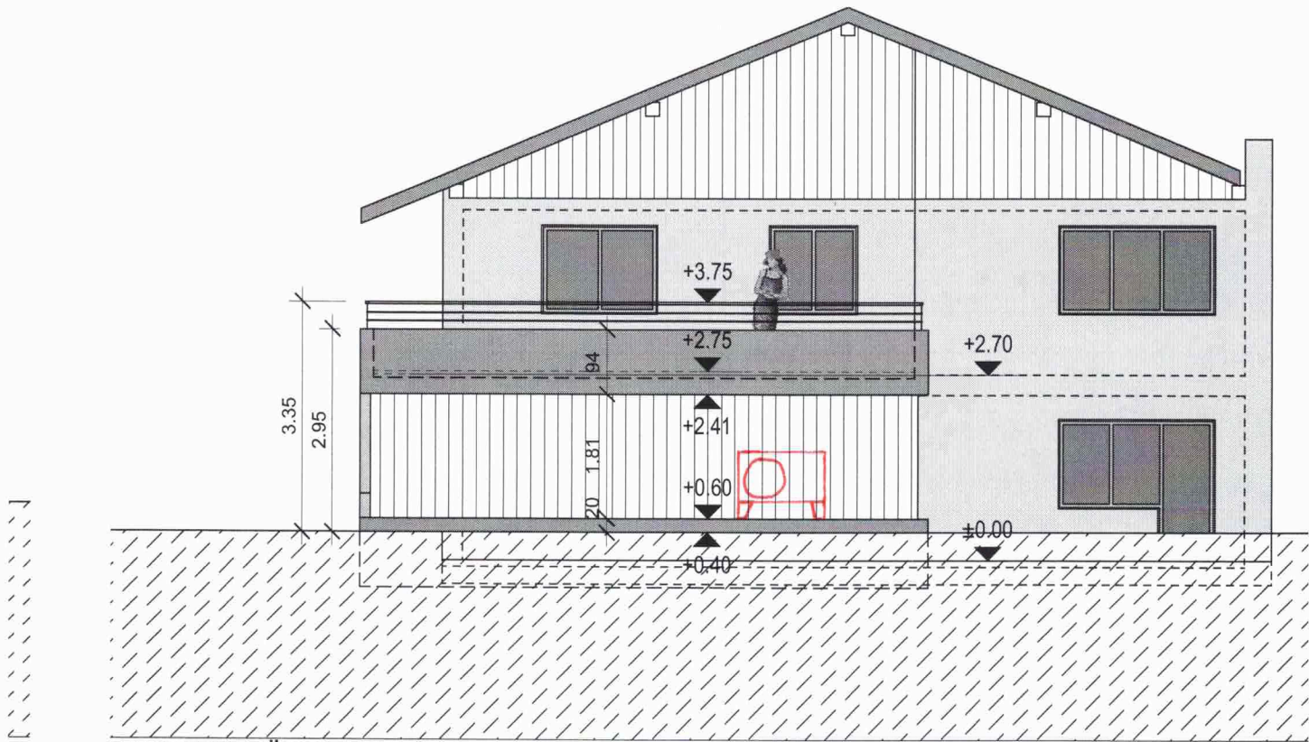
ANSICHT SÜD-WEST
