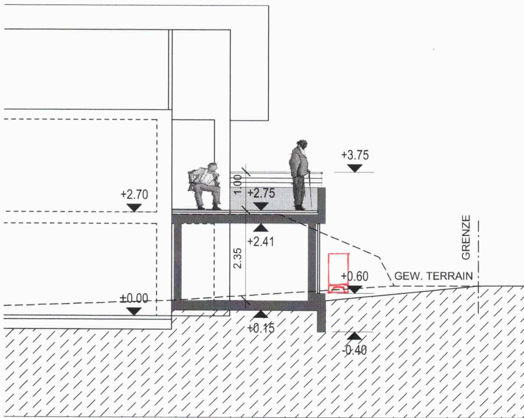
QUERSCHNITT
