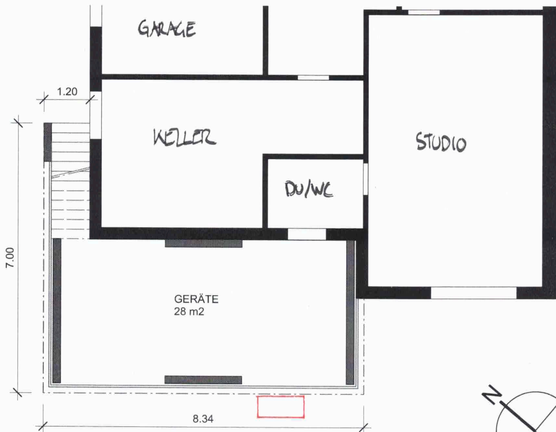
ERDGESCHOSS
