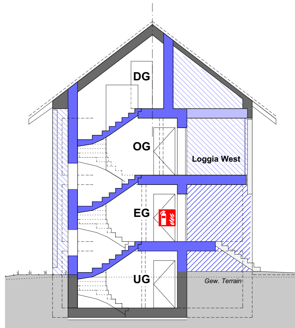
Schnitt B–B
