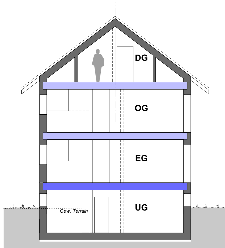
Schnitt A–A
