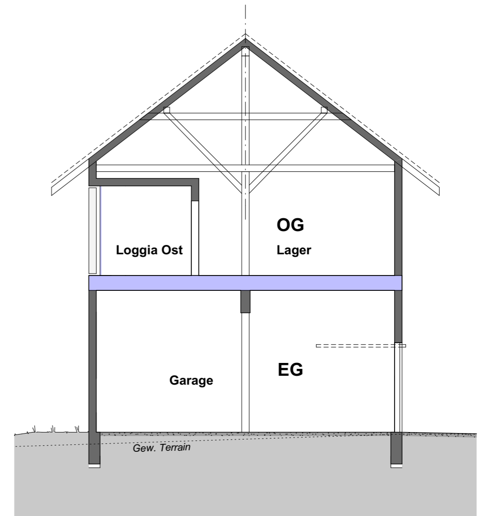
Schnitt C–C
